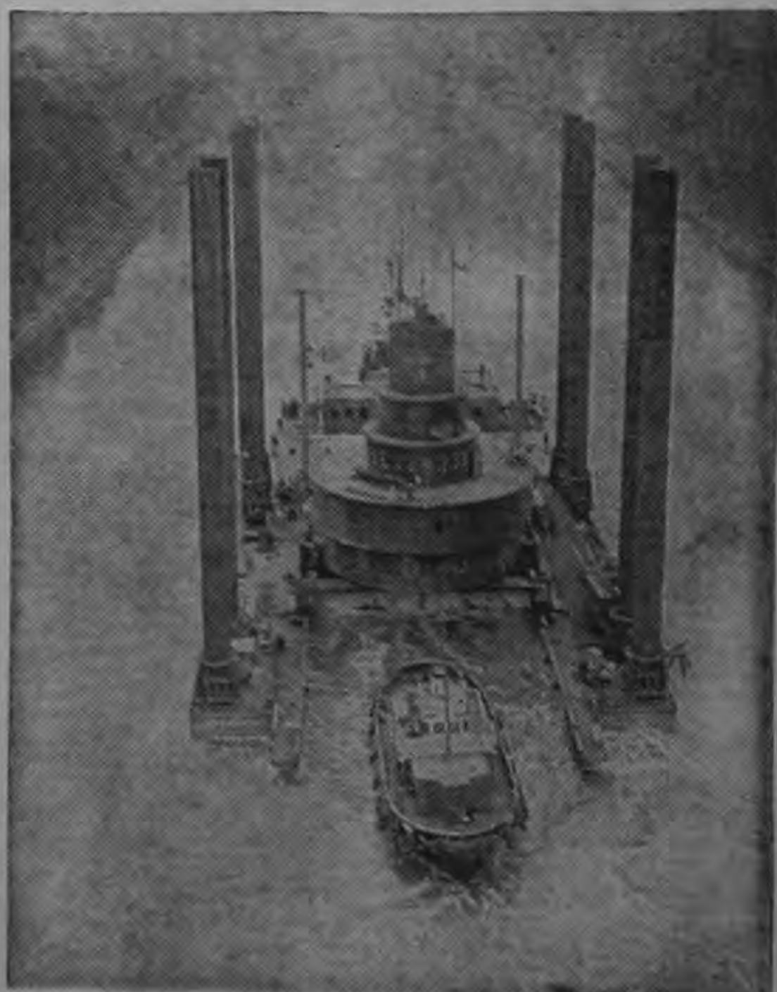
LA CUPULA DE UN FARO DE VIAJE. La cúpula del nuevo faro "Alte Weser" es transportada al mar del Norte. Este faro se encuentra en un punto importante en la cadena de radar que se está montando en la República Federal de Alemania en el bajo y en el exterior Weser. La cadena debe facilitar que incluso en tiempo brumoso puedan conducirse con seguridad los barcos hasta Bremen. Los remolcadores "Hoheweg" y "Stedingen" llevan la cúpula para el "Alte Weser" por el canal de Kiel al Weser. En la cúpula, de 300 Tn de peso están las salas para la tripulación y las salas de trabajo y el fanal. El nuevo faro va a ser llamado "Roter Sand".
